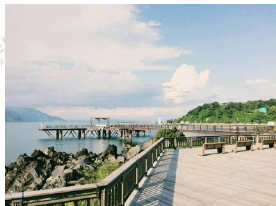
樱岛（活火山）
